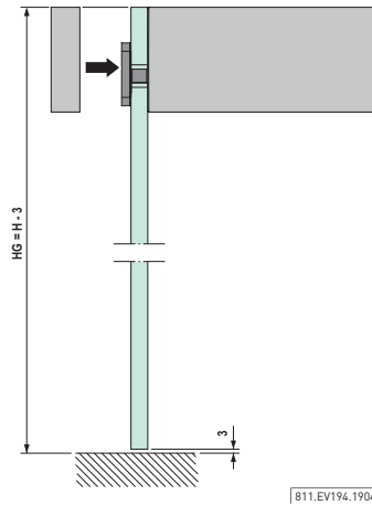
Situazioni di montaggio con supporto per parete in vetro
