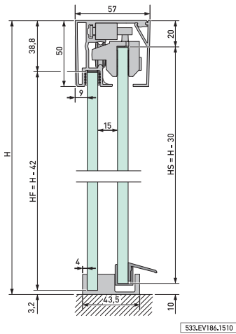
Situazioni di montaggio con profilo perimetrale
