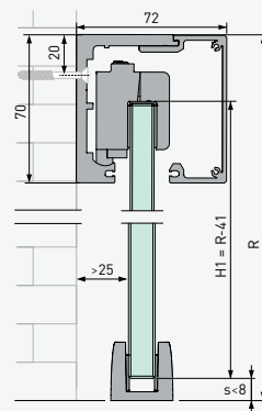
Systèmes avec deux vantaux sans vantail fixe
