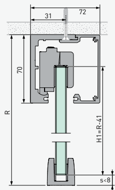
Systèmes avec un vantail sans vantail fixe
