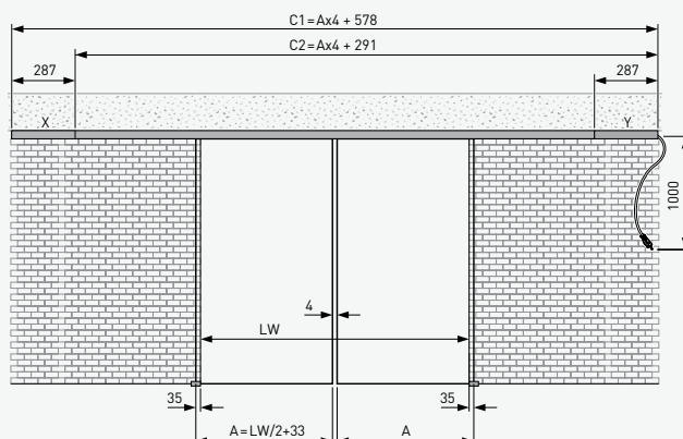
Systèmes avec deux vantaux sans vantail fixe
