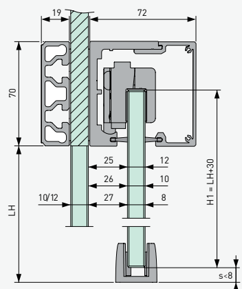
Montage sur façade vitrée
