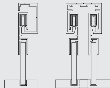
Herraje Penda
